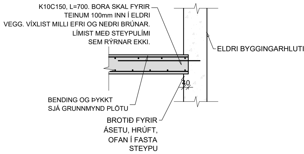
D Snið 1:20
