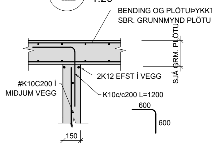
D Snið 1:20
