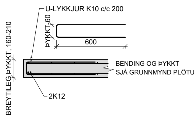
B Snið 1:20
